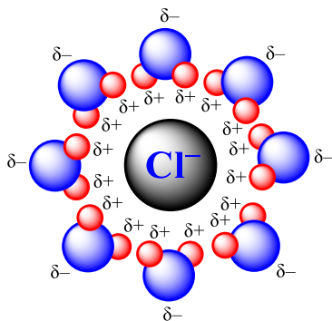
Рисунок 3 – Гидратация ионов
