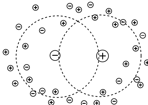
Рисунок 4 – Модель ионной атмосферы
