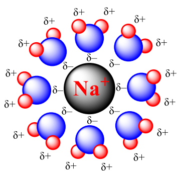
Рисунок 3 – Гидратация ионов
